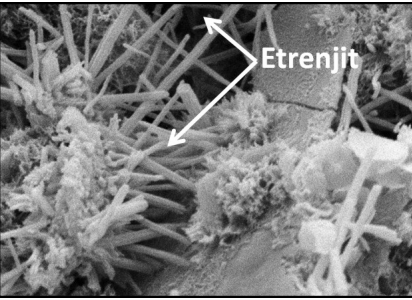
Şekil 12: Taramalı elektron mikroskopundan bakıldığında çimento hamurunda oluşan etrenjitlerin görünümü
